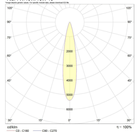
*Albi 7W/13W/18W 15°
