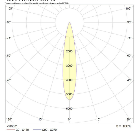
*Bron 7W/13W/18W 15°
