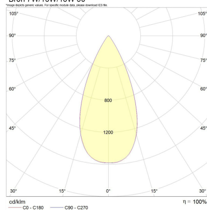
*Bron 7W/13W/18W 50°
