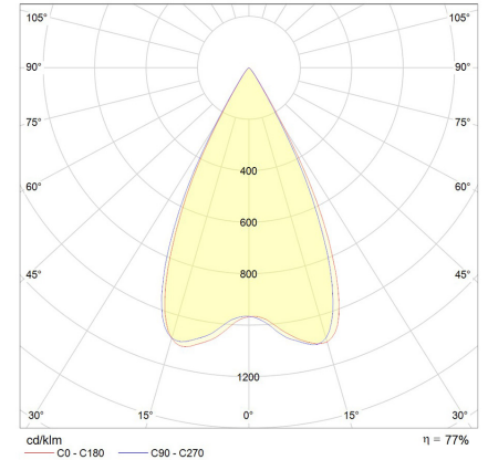
Cannes Maxi Pendant 40°
