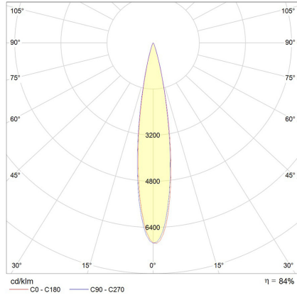
Cannes Maxi Pendant 16°
