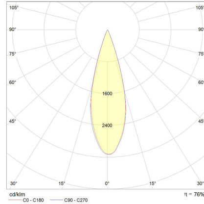
Cannes Maxi Pendant 29°
